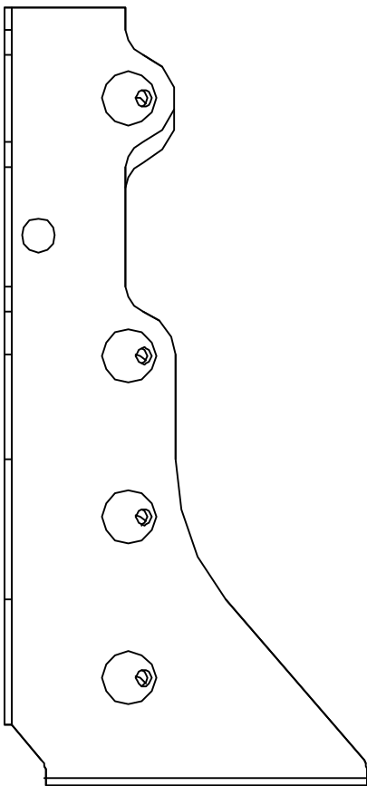
HUS28 - LEFT SIDE VIEW
