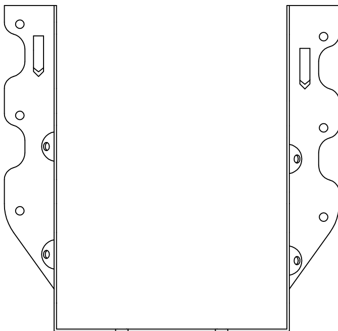
JUS28-3 -FRONT VIEW
