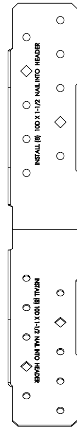
CSH-TZ-FRONT-VIEW
